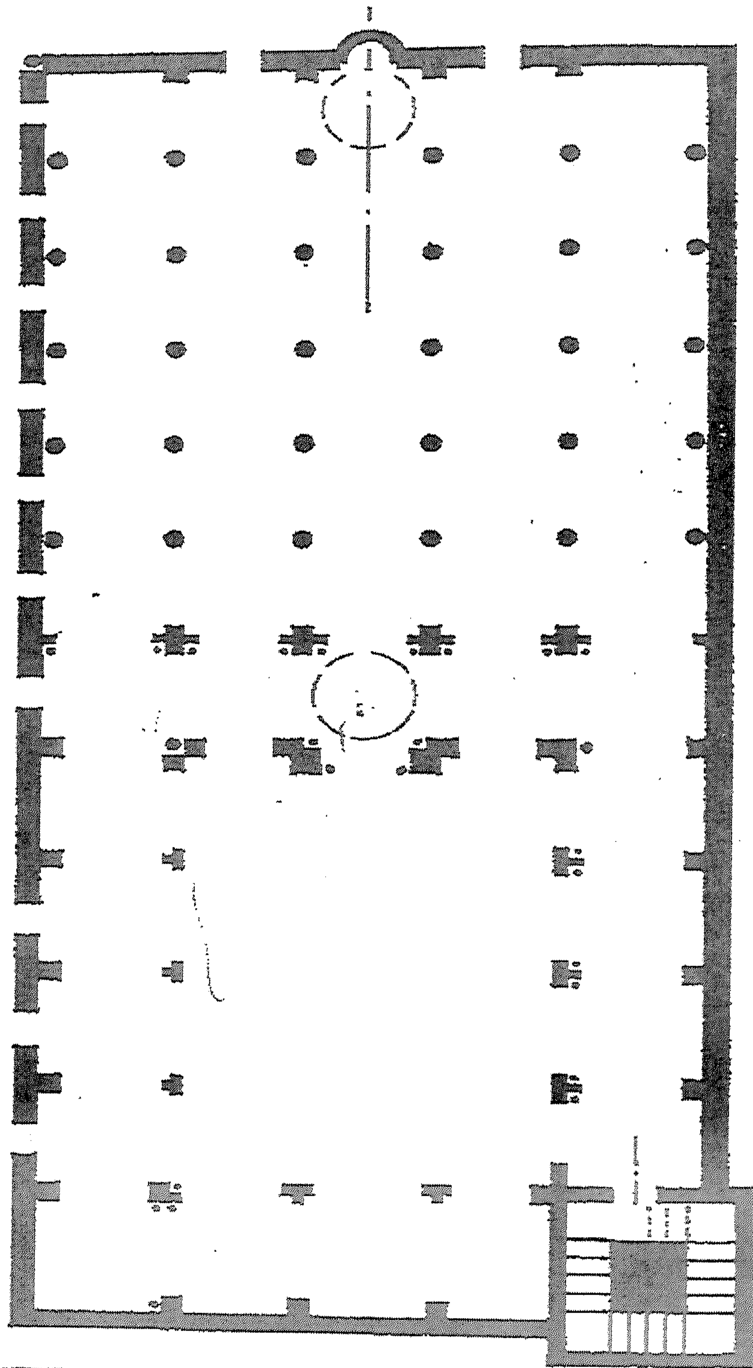
(شكل رقم ٤١) رسم تخطيطي لجامع صفاقس في نهاية القرن الرابع الهجري / العاشر الميلادي عن ليزين
